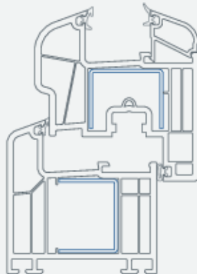
Arcade s predsadeným krídlom
