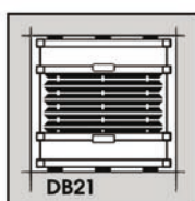
DB21 Max. šířka 100 cm Max. výška 250 cm
